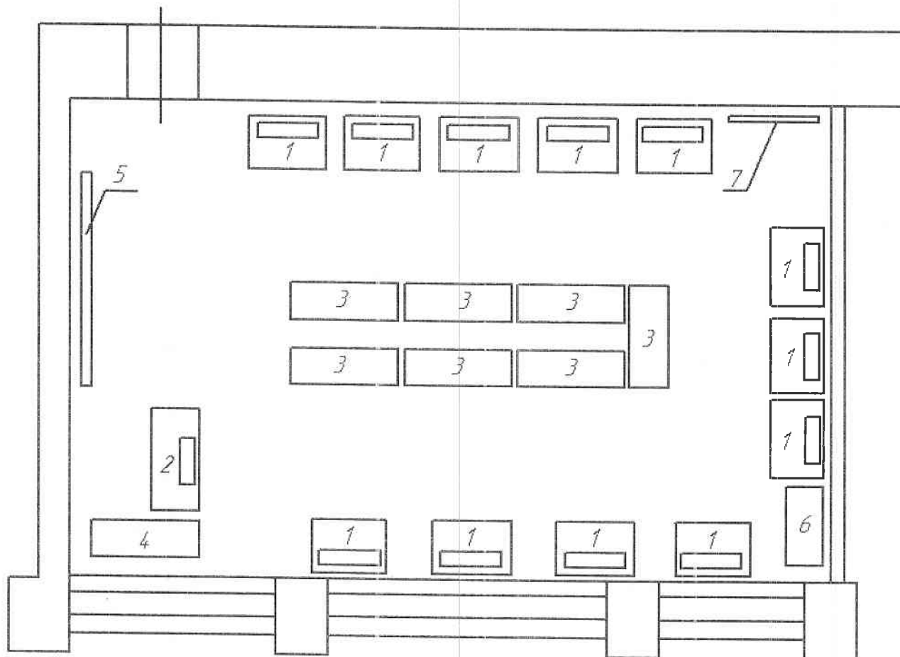
Схема расположения стационарного оборудования, приборов и установок кабинета (лаборатории)
